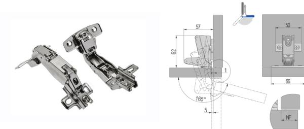
Петля мебельная GTV 165°
