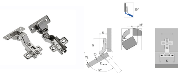
Петля мебельная GTV 30° угловая
