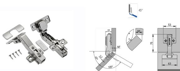
Петля мебельная GTV 45° угловая с доводчиком
