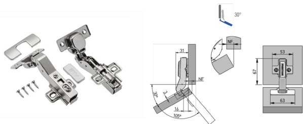
Петля мебельная GTV 30° угловая с доводчиком
