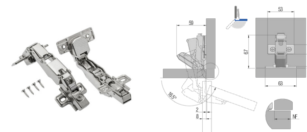
Петля мебельная GTV 165° с доводчиком
