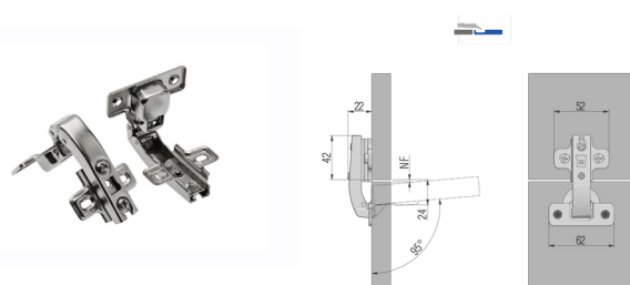
Петля мебельная GTV 90° под фальшпанель
