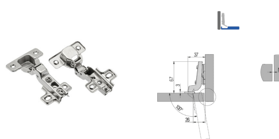
Петля мебельная GTV 93° вкладная
