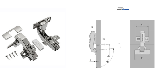
Петля мебельная GTV 97° под фальшпанель с доводчиком
