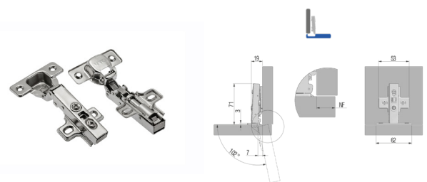
Петля мебельная GTV 102° накладная с доводчиком
