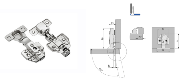
Петля мебельная GTV 95° PRESTIGE накладная с доводчиком
