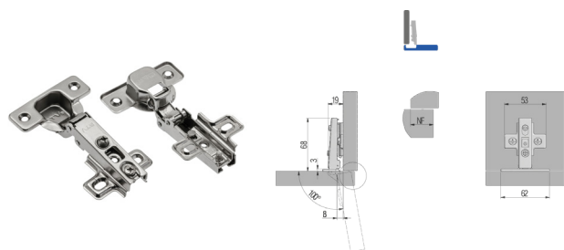
Петля мебельная GTV 93° накладная
