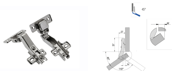
Петля мебельная GTV 45° угловая
