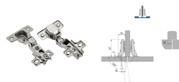
Петля мебельная GTV 100° полунакладная
