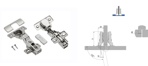
Петля мебельная GTV 102° полунакладная с доводчиком
