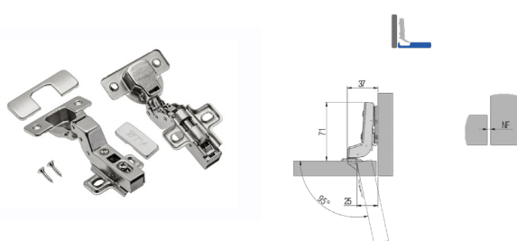
Петля мебельная GTV 102° вкладная с доводчиком
